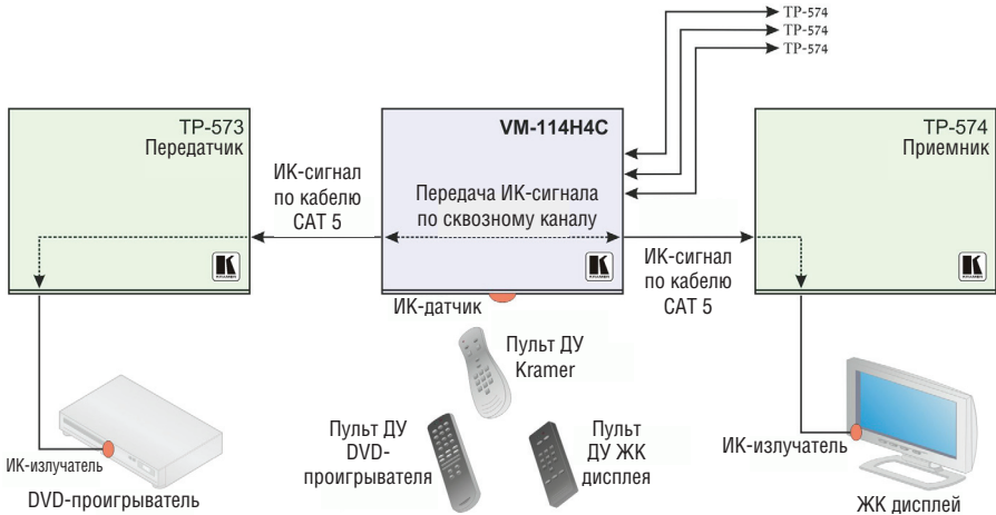
Рис. 5. Локальное ИК-управление VM-114H4C и передача сигнала по сквозному каналу — пример 1
