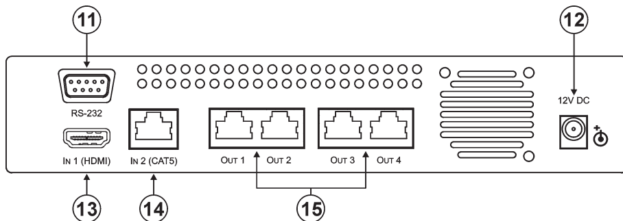
Рис. 2. Задняя панель VM-114H4C
