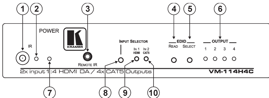
Рис. 1. Передняя панель VM-114H4C
