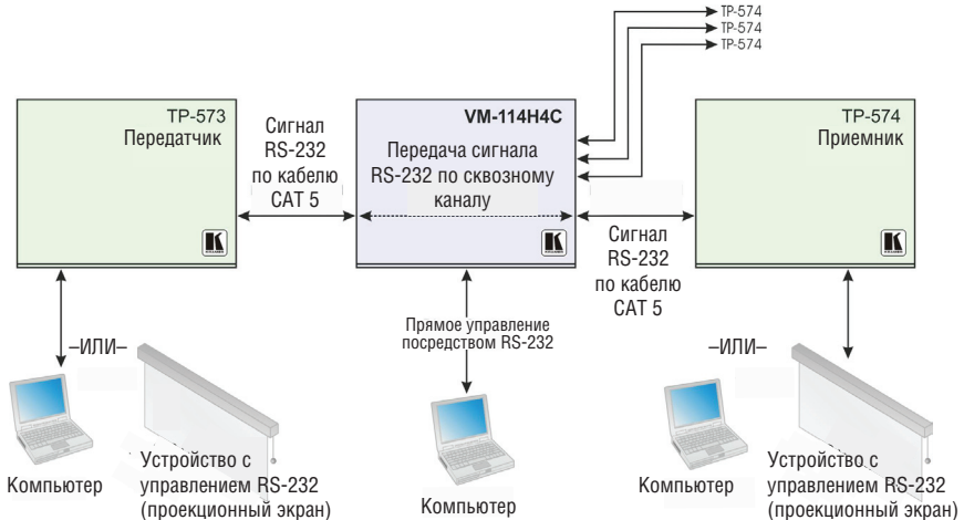
Рис. 4. Управление VM-114H4C посредством RS-232 и передача сигнала по сквозному каналу
