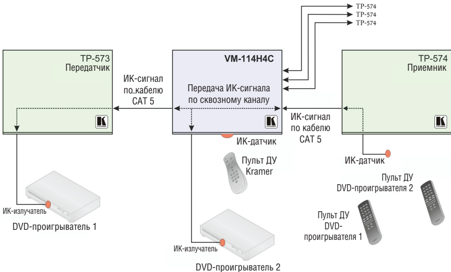
Рис. 7. Локальное ИК-управление VM-114H4C и передача сигнала по сквозному каналу — пример 3
