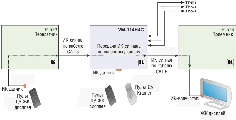
Рис. 6. Локальное ИК-управление VM-114H4C и передача сигнала по сквозному каналу — пример 2
