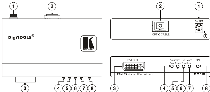
Рис. 2. Передняя панель оптического приемника DVI 671R
