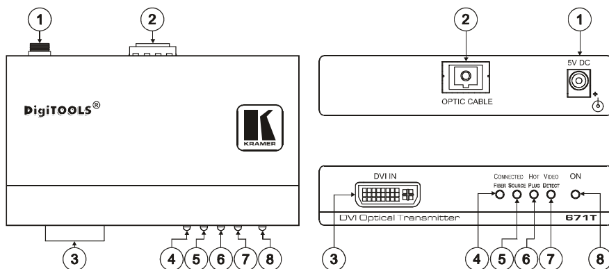
Рис. 1. Передняя панель оптического передатчика DVI 671T
