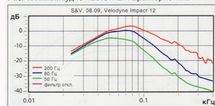
Рис. 1. Амплитудно-частотная характеристика
